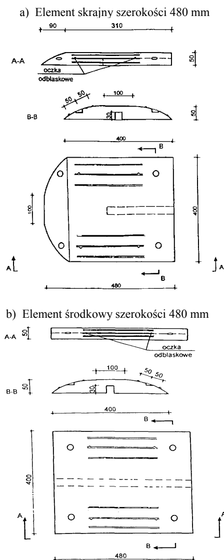
Rys. 2. Próg typu listwowego długości 400 mm i wysokości 50 mm
