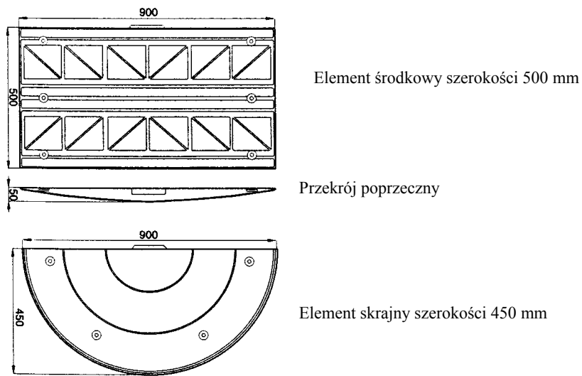
Rys. 4. Przykład umocowania progu do nawierzchni jezdni
