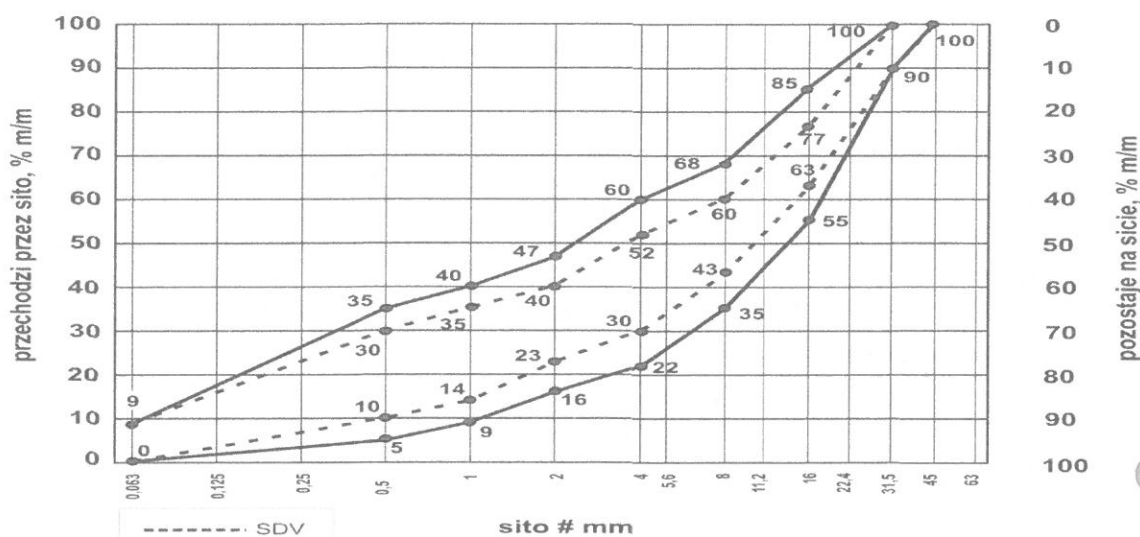
Rysunek 1. Obszar uziarnienia optymalnych mieszanek żwirowych 0/31,5
