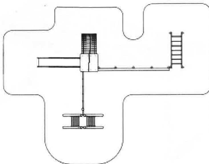
Rys. nr 8. Zestaw zabawowy - widok strefy bezpieczeństwa
